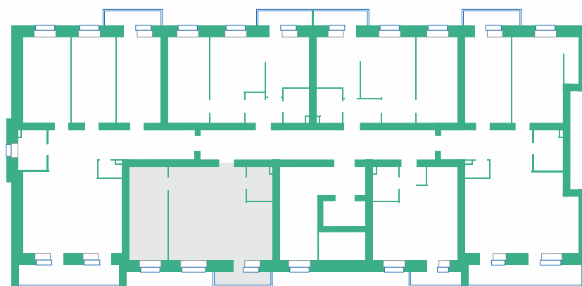
Планировка этажа
