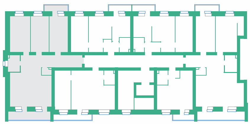
Планировка этажа
