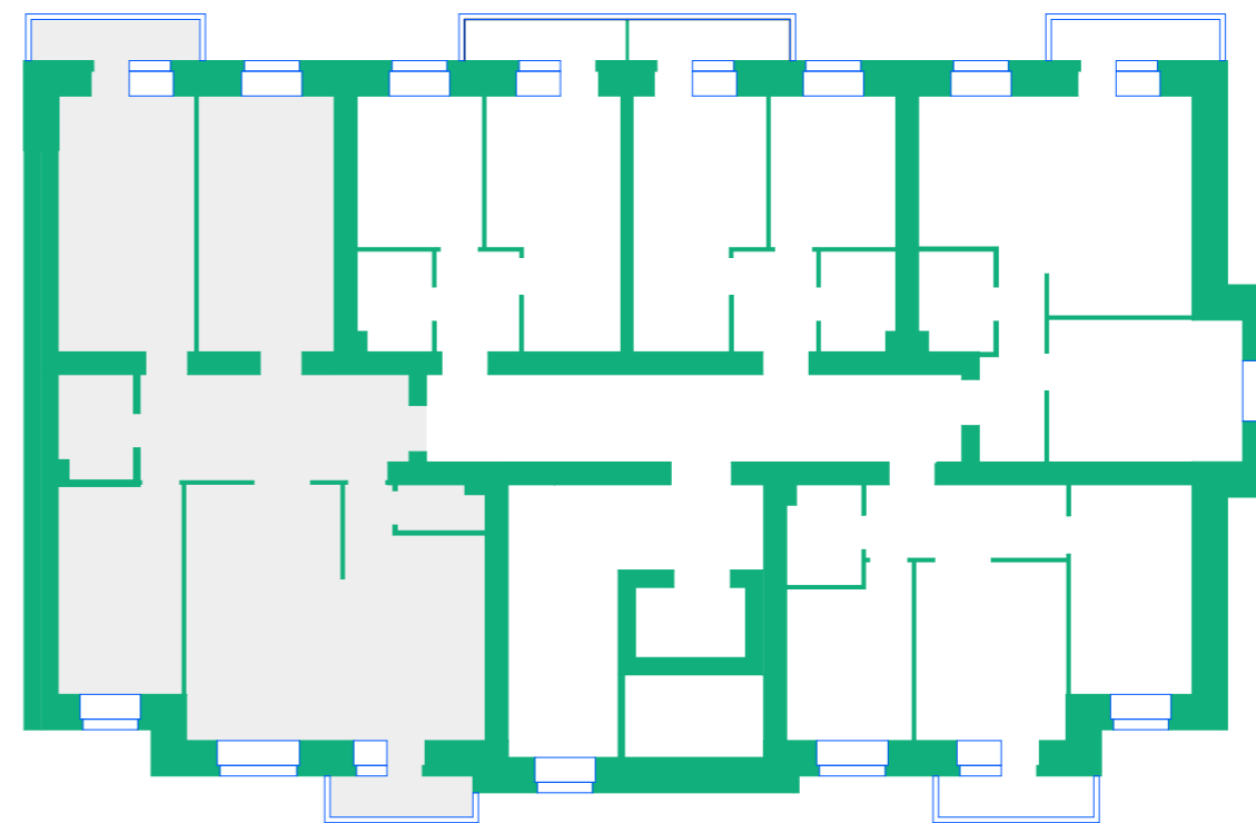
Планировка этажа
